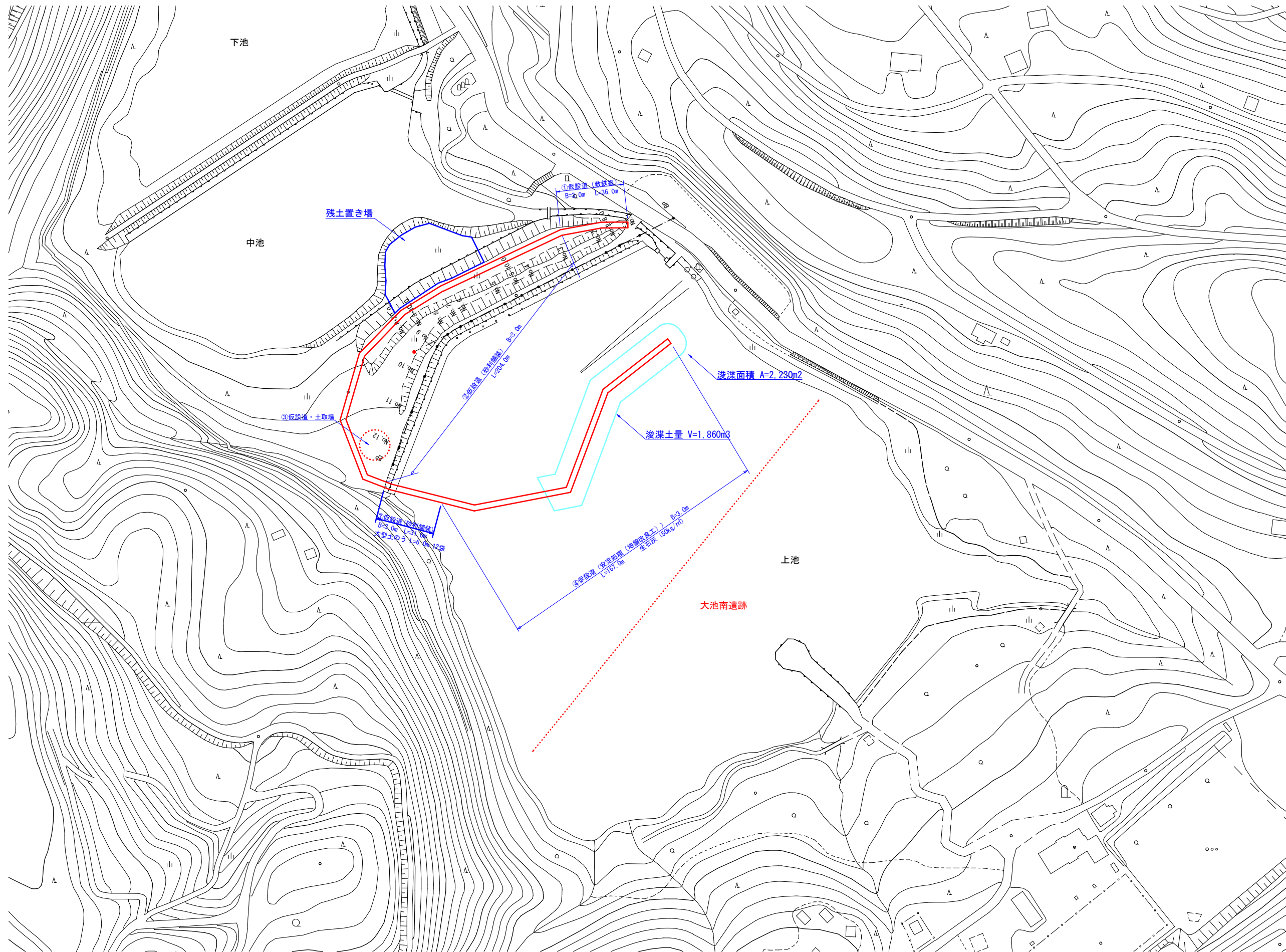
仮設工平面図 S=1/1000
