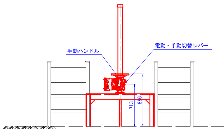
C-C 矢視 (S=1:20)
