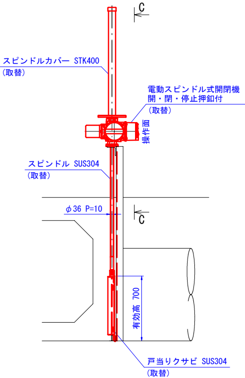
B-B 矢視 (S=1:20)
