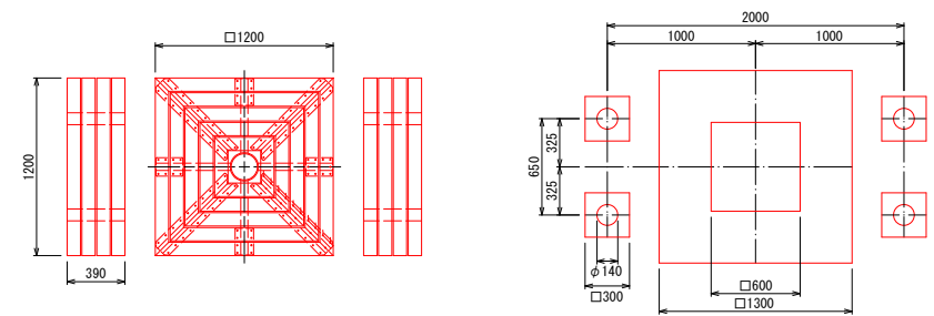
基礎伏せ図 S=1:20 (A3 S=1:40)
