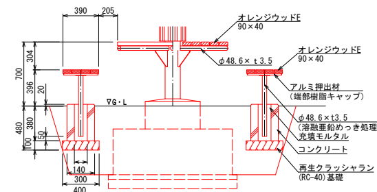
ベンチ詳細図 S=1:20 (A3 S=1:40)
