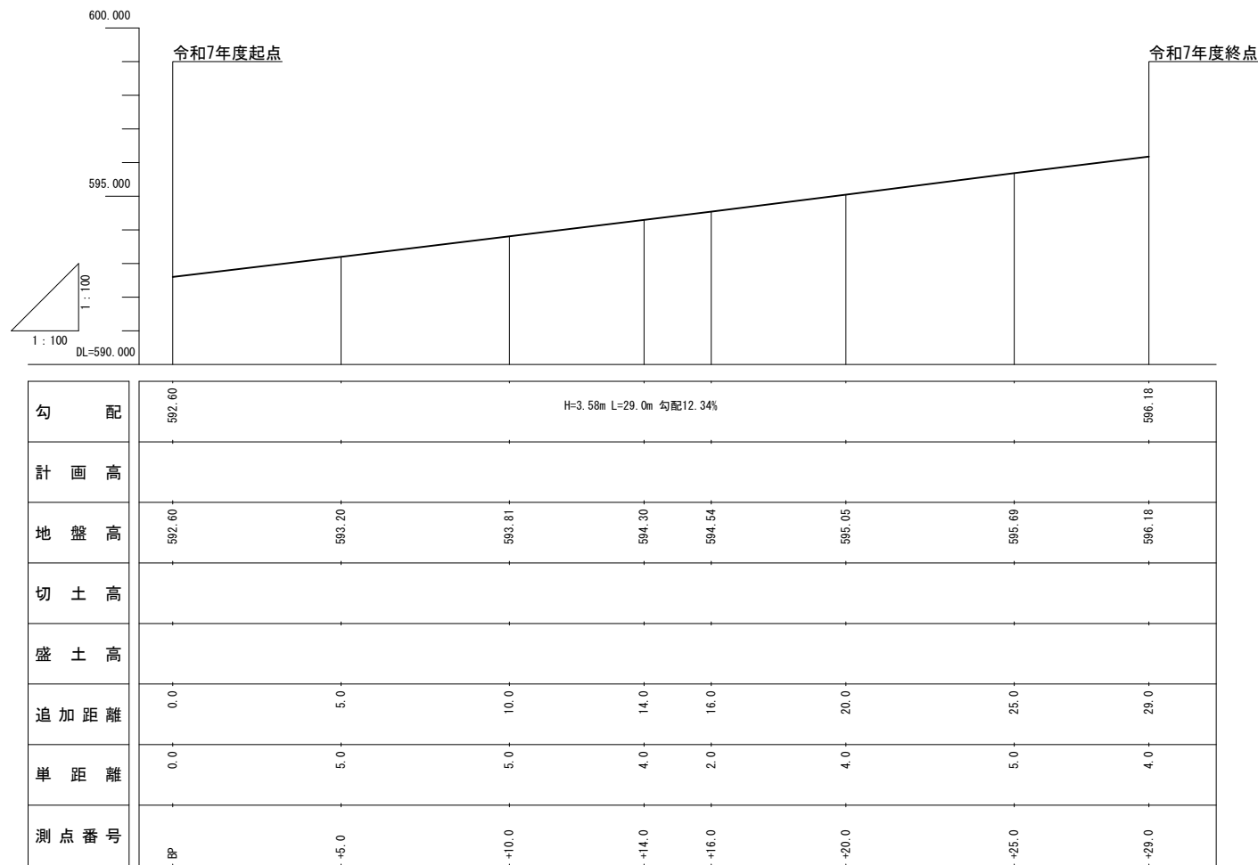
縦 断 図 S=1/100
