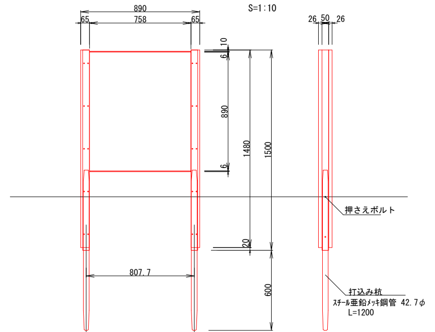
案内看板構造図 (アコヤAWS (打込み杭仕様) 同等品以上) (参考図)
