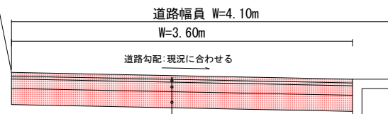
舗装標準断面図
