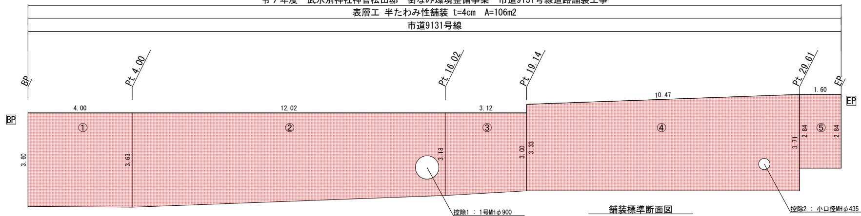
舗装標準断面図
