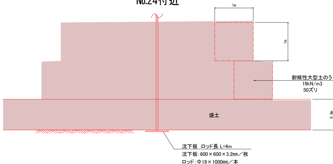
構造図（参考図） No.24付近
