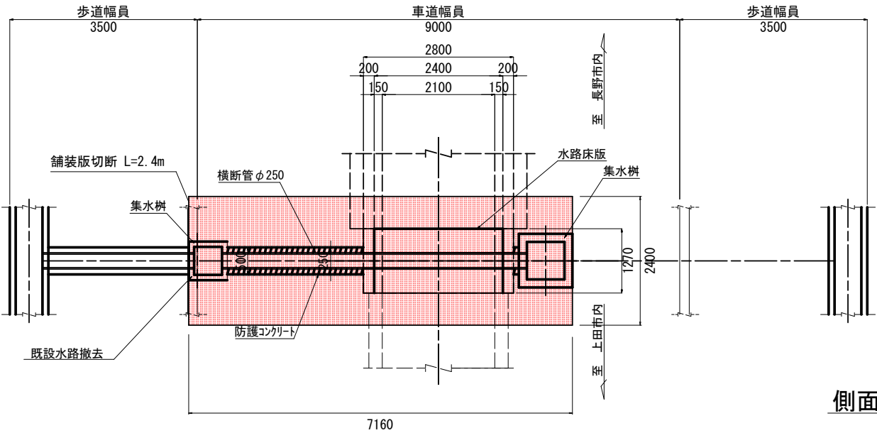
平面図 S=1/50
