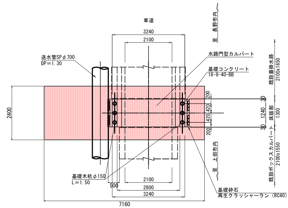
平面図 S=1/50
