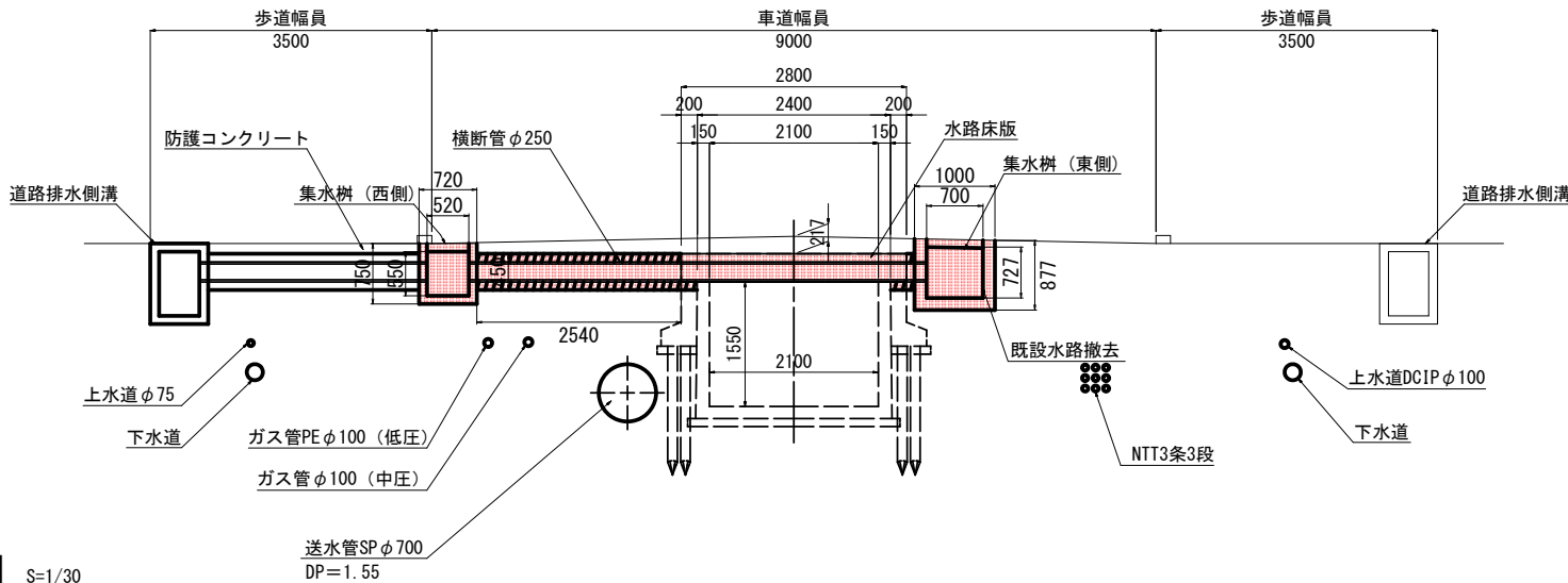
側面図 S=1/30
