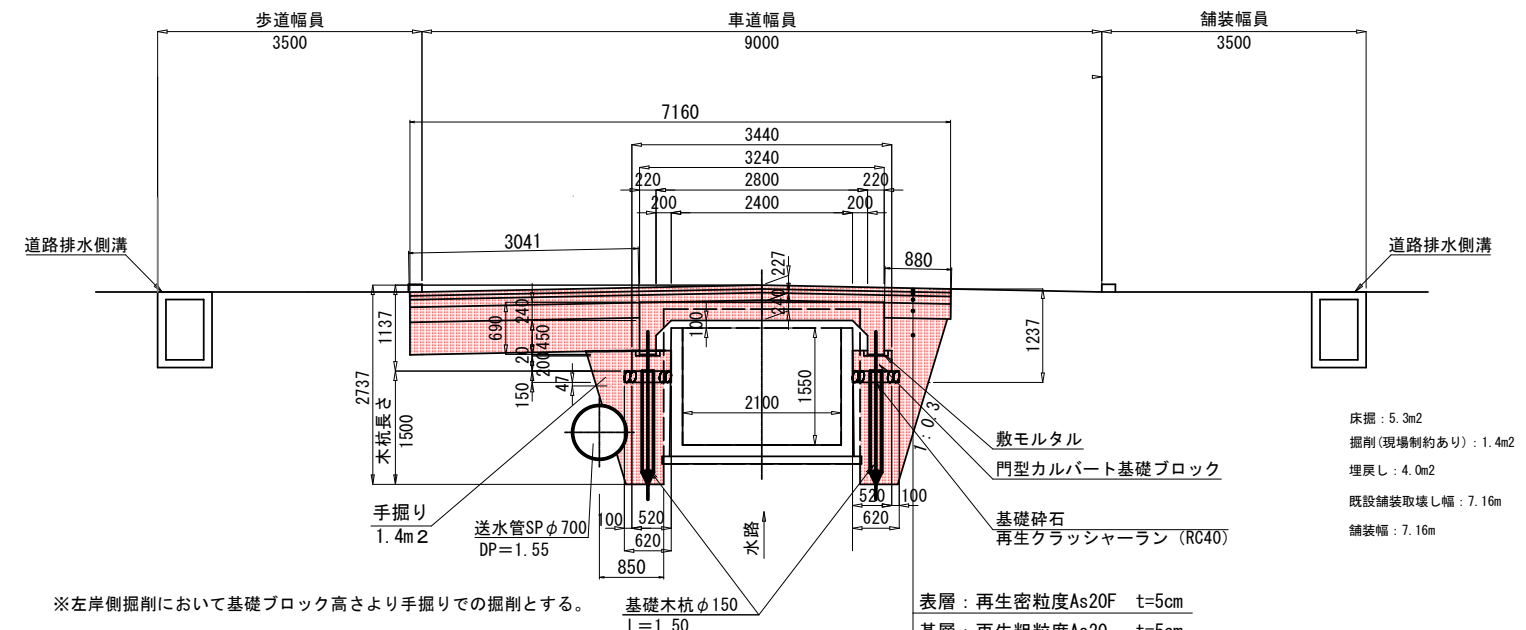
標準横断面図 S=1/50
