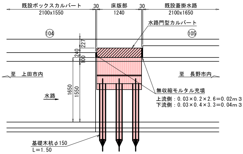
側面図 S=1/30
