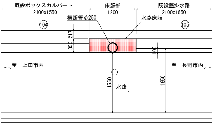
側面図 S=1/30
