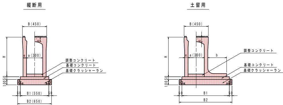
自由勾配側溝 (参考図)
