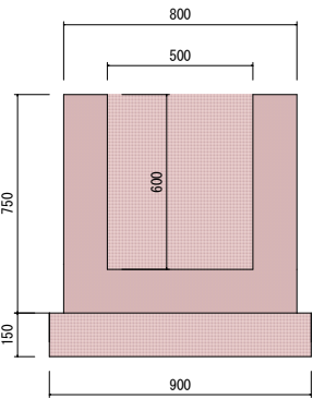
集水樹 500×500 H=600
