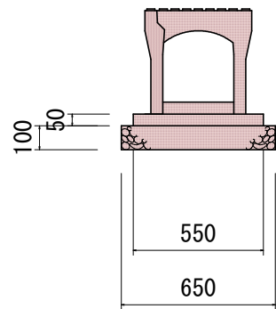
自由勾配側溝構（縦断用） S=1/10 参考図
