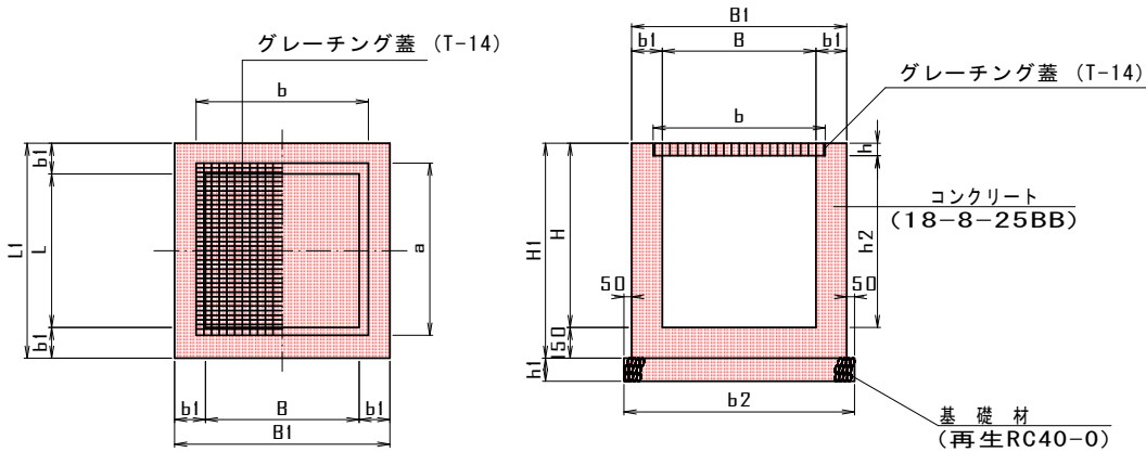
集水樹 寸法表
