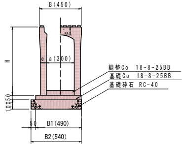
自由勾配側溝（縦断用）300×600～700 （参考図）
