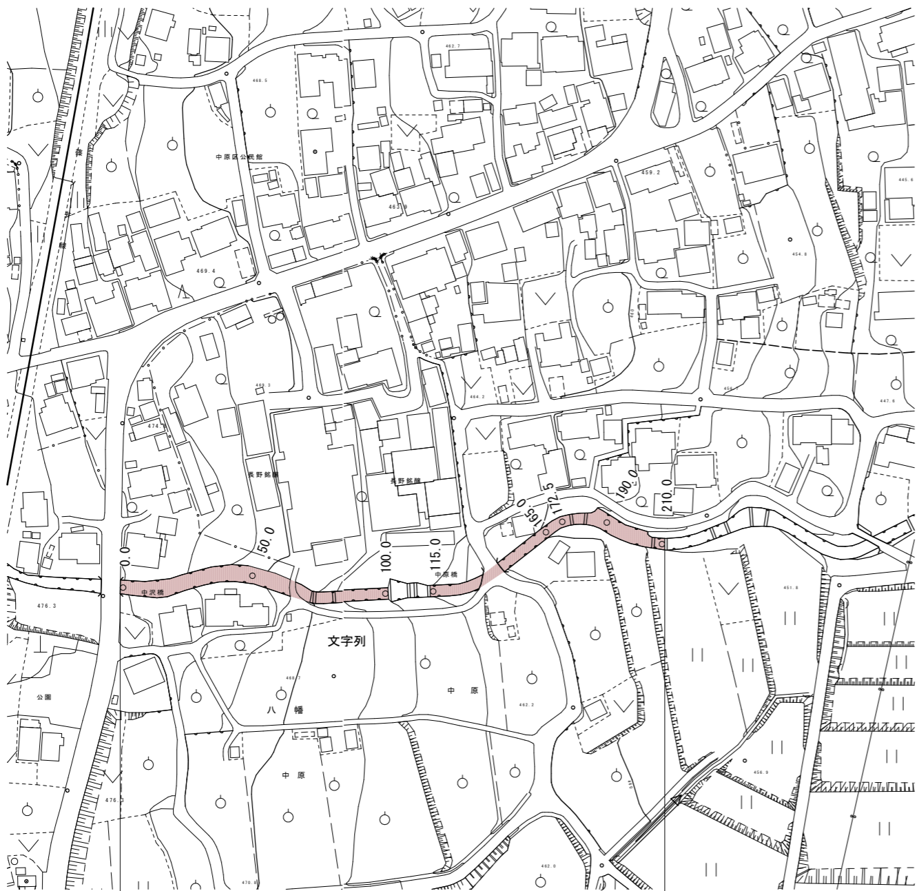
平面図 S=1:1000
