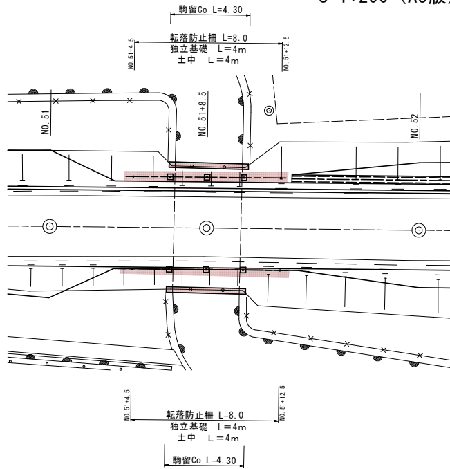
平面図
