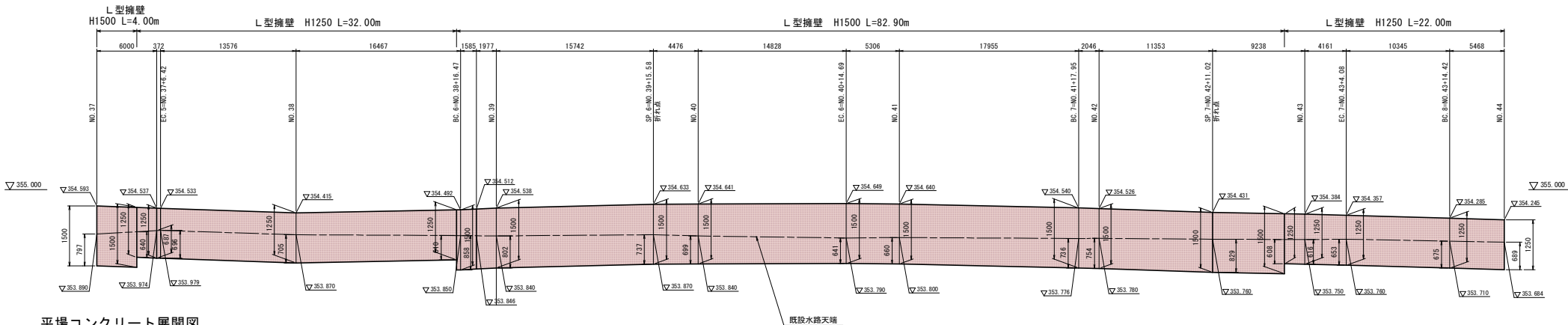
平場コンクリート展開図
