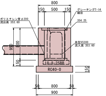
B-B断面
