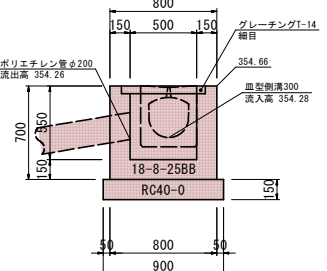
B-B断面
