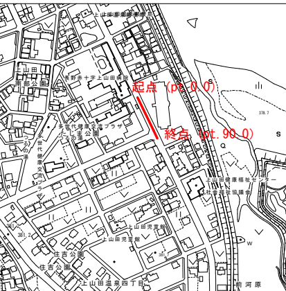
位置図 S=1:5000
