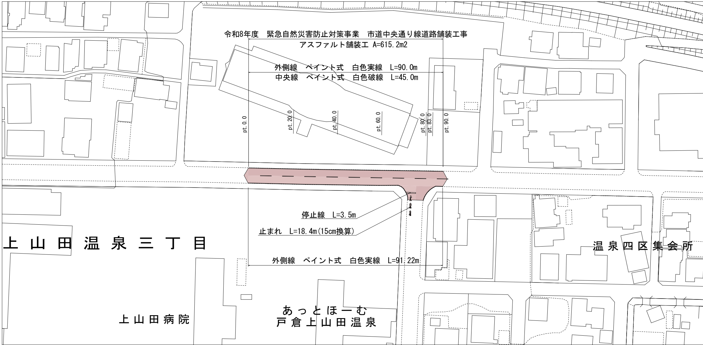
平面図 S=1:500
