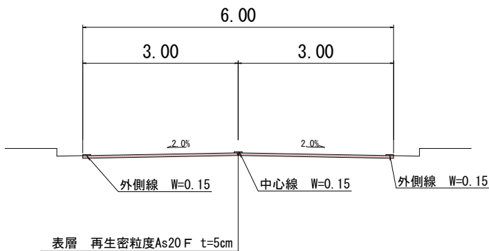
本線横断面図
