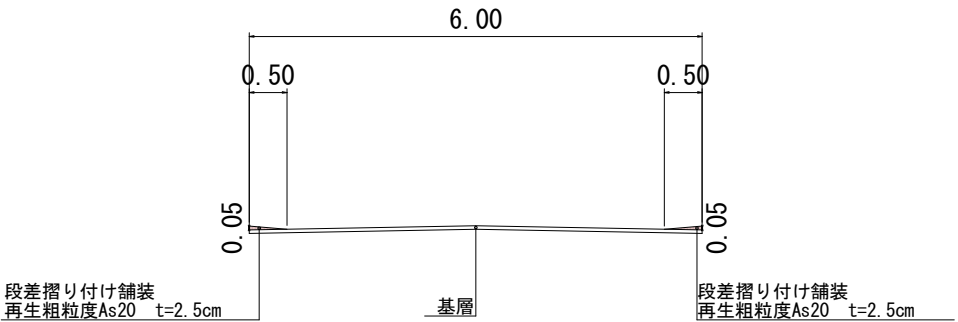
段差摺り付け舗装横断面図
