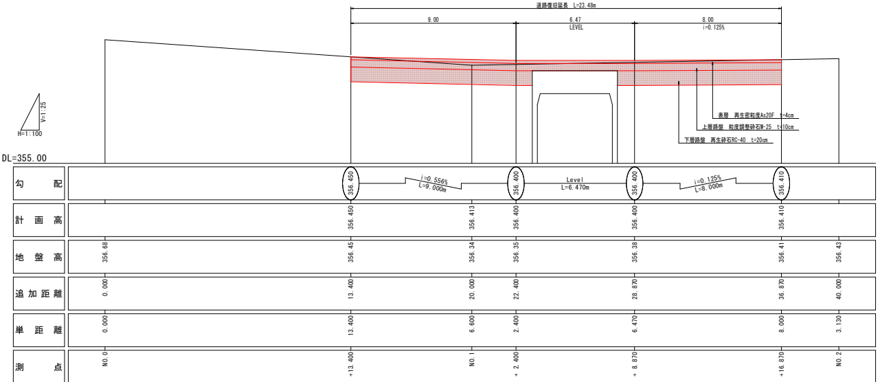
縦断面 SH=1:100, SV=1:25
