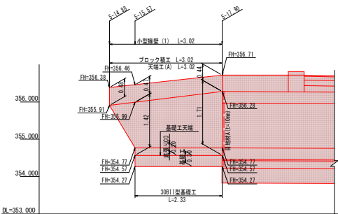
上流左岸取付護岸工展開図 S=1:50
