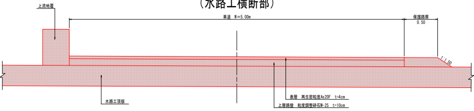
標準横断面 (水路工横断面) S=1:20
