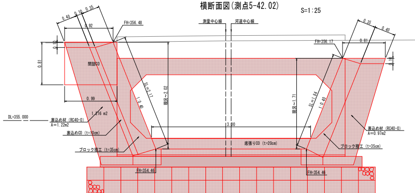
下流側ブロック積護岸工 横断面図(測点5-42.02) S=1:25
