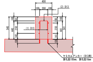
断面图 ( 4 - 4 )
