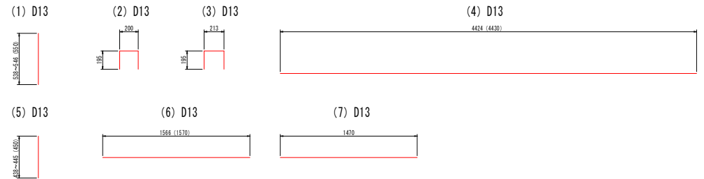
地覆鉄筋加工図 S=1:20
