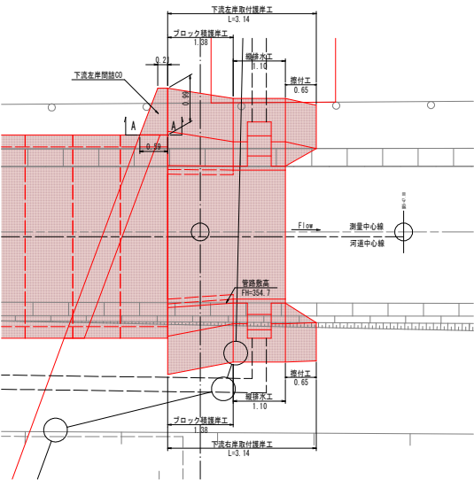
下流側平面図 S=1:50
