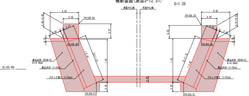
上流側ブロック積護岸工 横断面図 (測点5-12.51)
