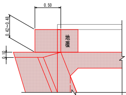
断面図 S=1:25
