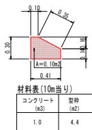
30B1型基礎工 (18-8-40BB) S=1:25
