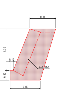
目地材E S=1:25
