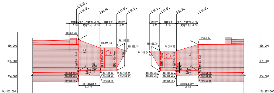
下流側ブロック積護岸工 横断面図(測点5-42.02) S=1:25
