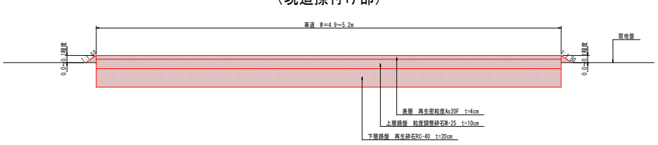
標準横断面 (現道擦付け部) S=1:20
