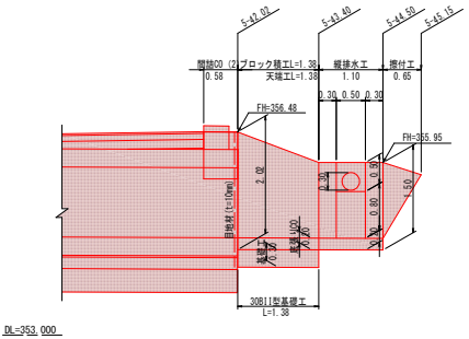
左岸側縦排水工展開図 S=1:50
