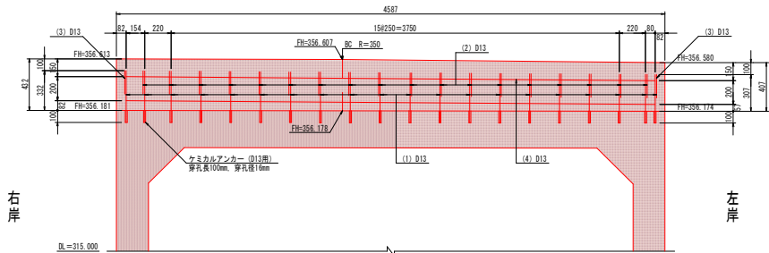
平面図 S=1:20
