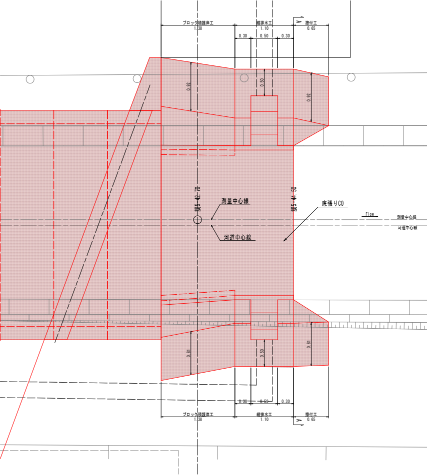
縦排水工平面図 S=1:25
