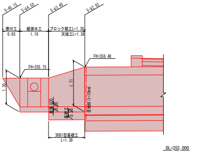
右岸側縦排水工展開図 S=1:50
