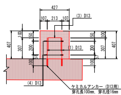
断面図 (5-5)
