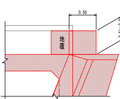
断面図 S=1:25
