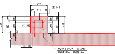
断面図 (3-3)
