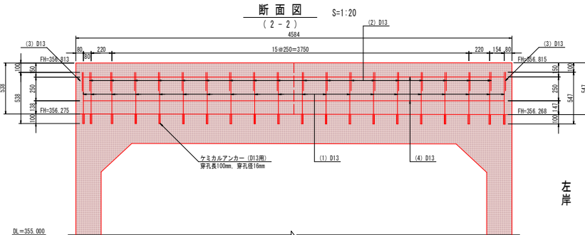
断面图 S=1:20
