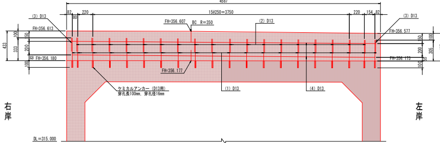
断面図 (2-2)
