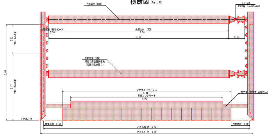
横断面図 S=1:20
