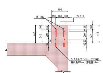
断面图 S=1:20 (7-7)
