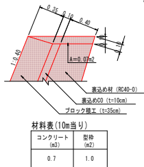
天端工 (A) S=1:25
