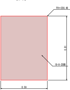
断面図 (A-A)
