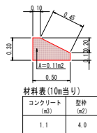
30B1型基礎工 (18-8-40BB) S=1:25
