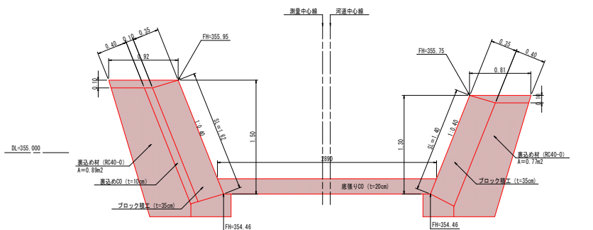
下流側ブロック積護岸工 横断面図(測点5-43.40) S=1:25
