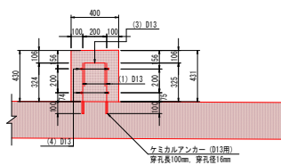
断面図 (4-4)
