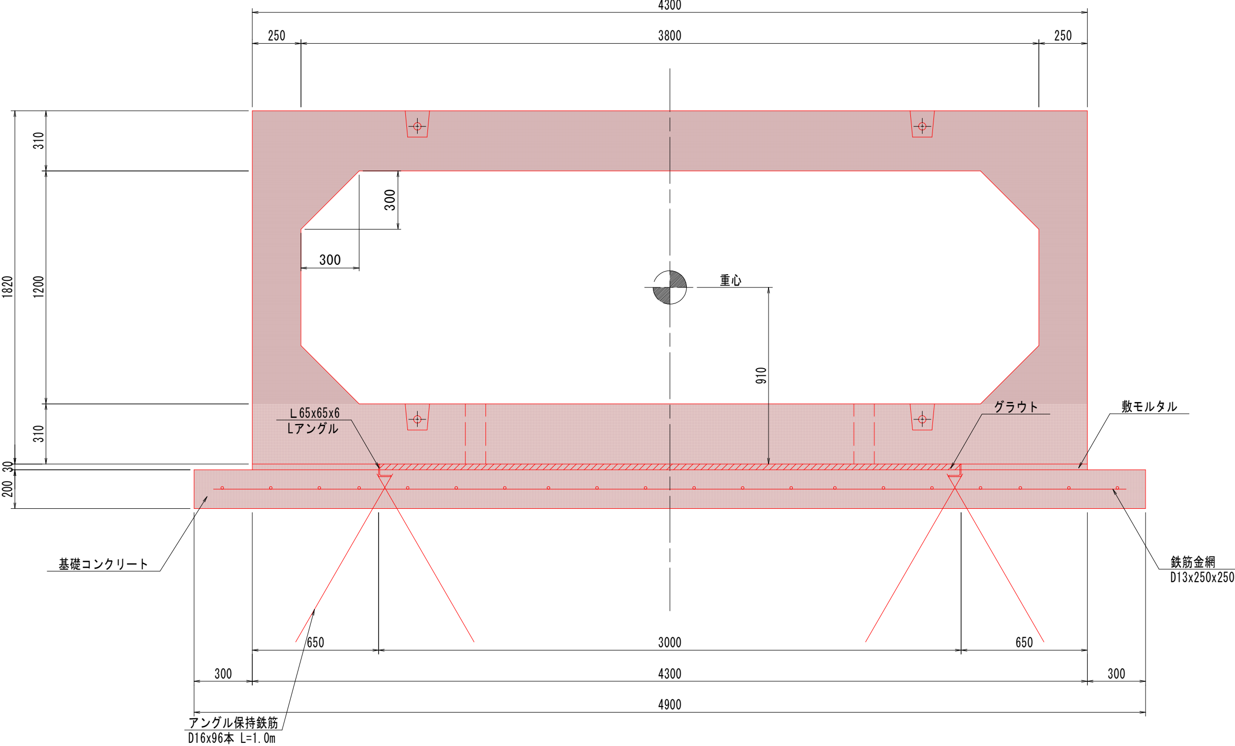
横断面 S=1:2
