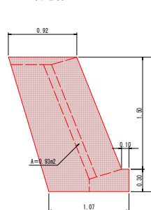
目地材D S=1:25
