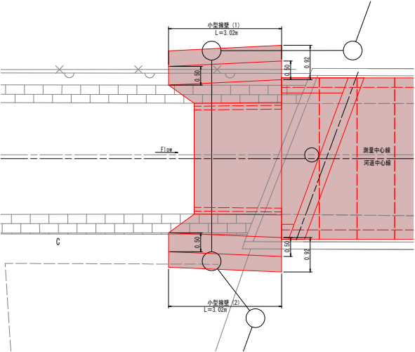
下流側平面図 S=1:50
