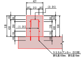
断面图 S=1:20 (6-6)
