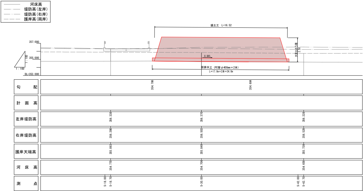
縦断面図 S=1:100
