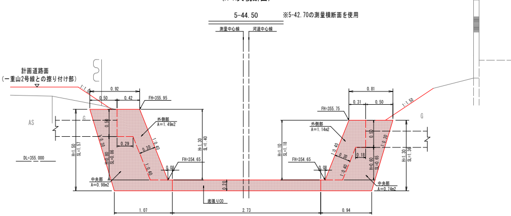
縦排水工横断面図 S=1:25
