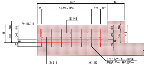
断面图 S=1:20 (6-6)
