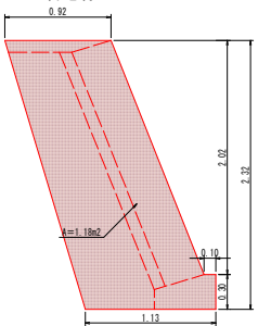
目地材B S=1:25
