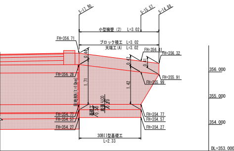
上流右岸取付護岸工展開図 S=1:50
