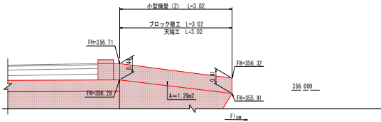
断面図 S=1:25
