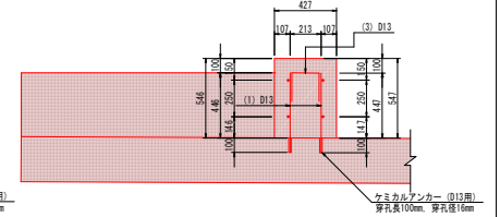
断面图 S=1:20 (7-7)
