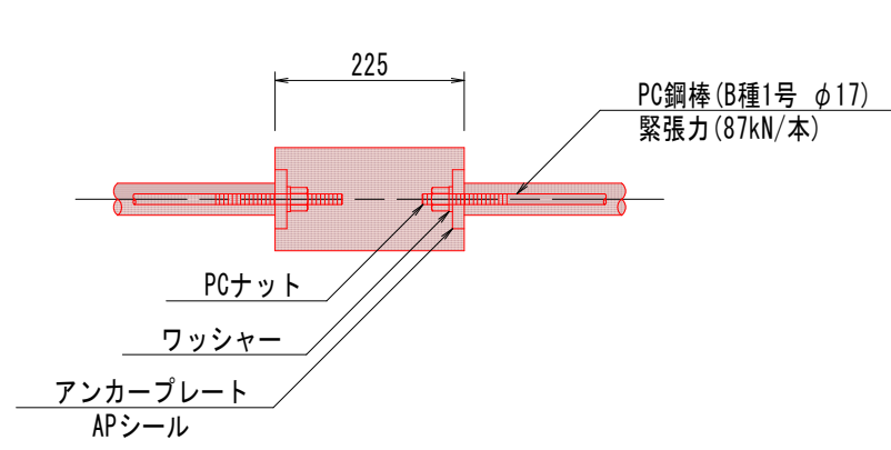
PC縦締め詳細図 S=1:10
