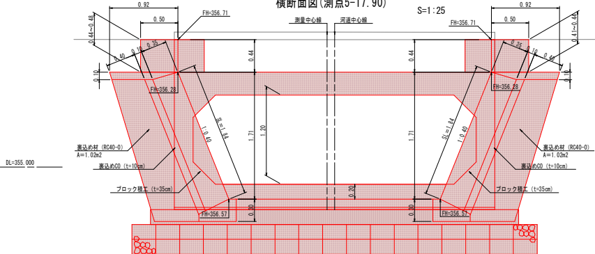
上流側ブロック積護岸工 横断面図 (測点5-17.90)
