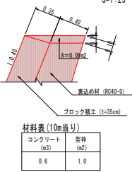
天端工 (B) S=1:25
