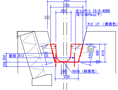
C-C断面 (帯工Ⅱ型)
