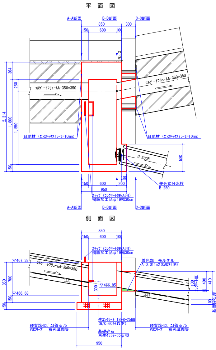
平面図
