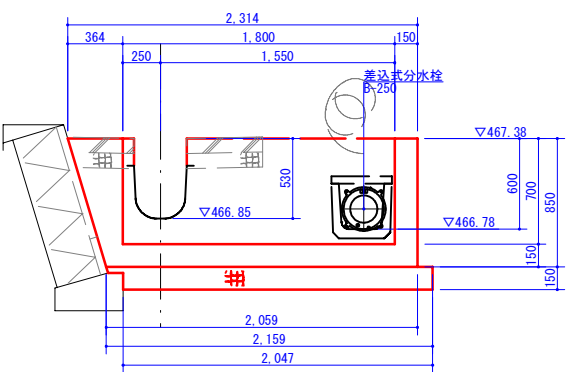
B-B断面
