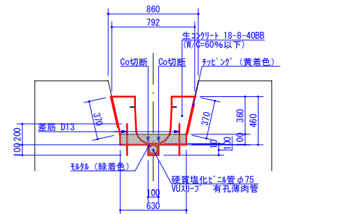
断面図
