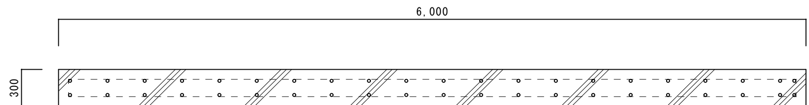
GHP架台基礎平面図1/30
