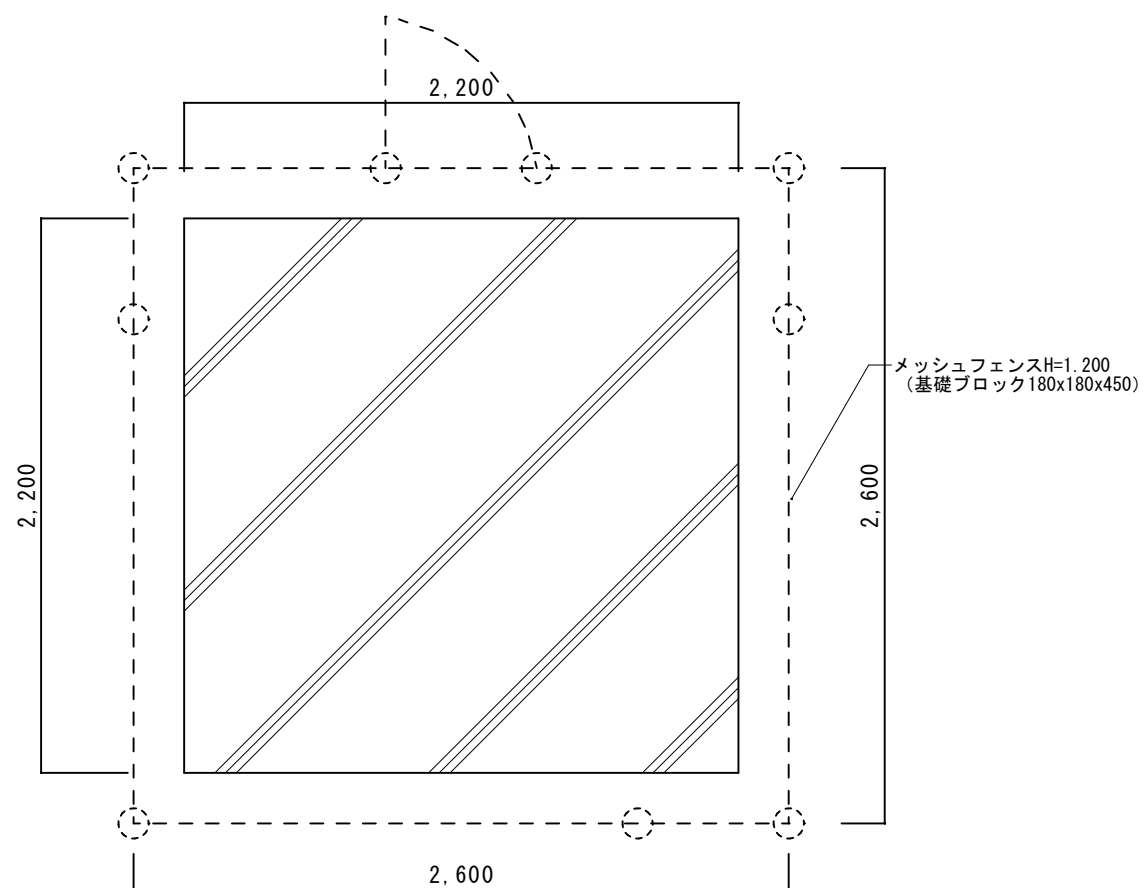
バルク基礎平面図1/30
