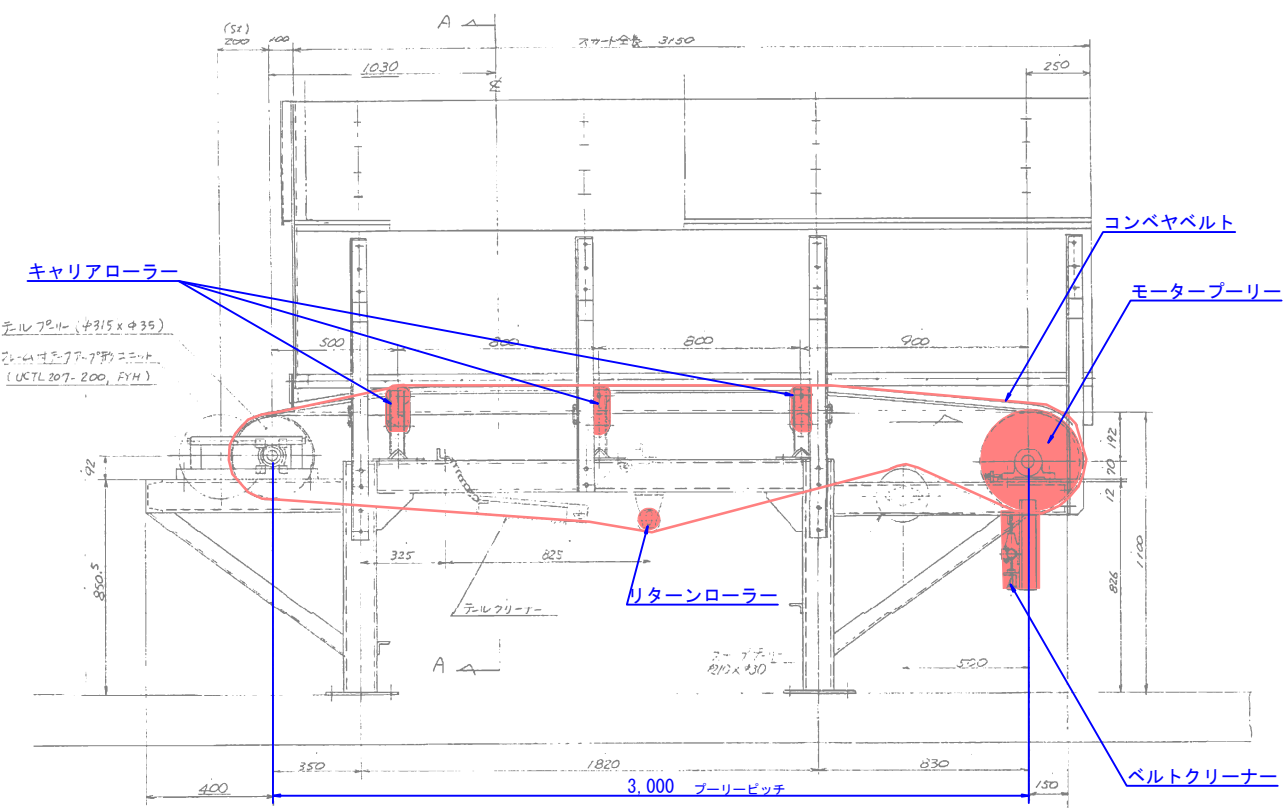
側面図
