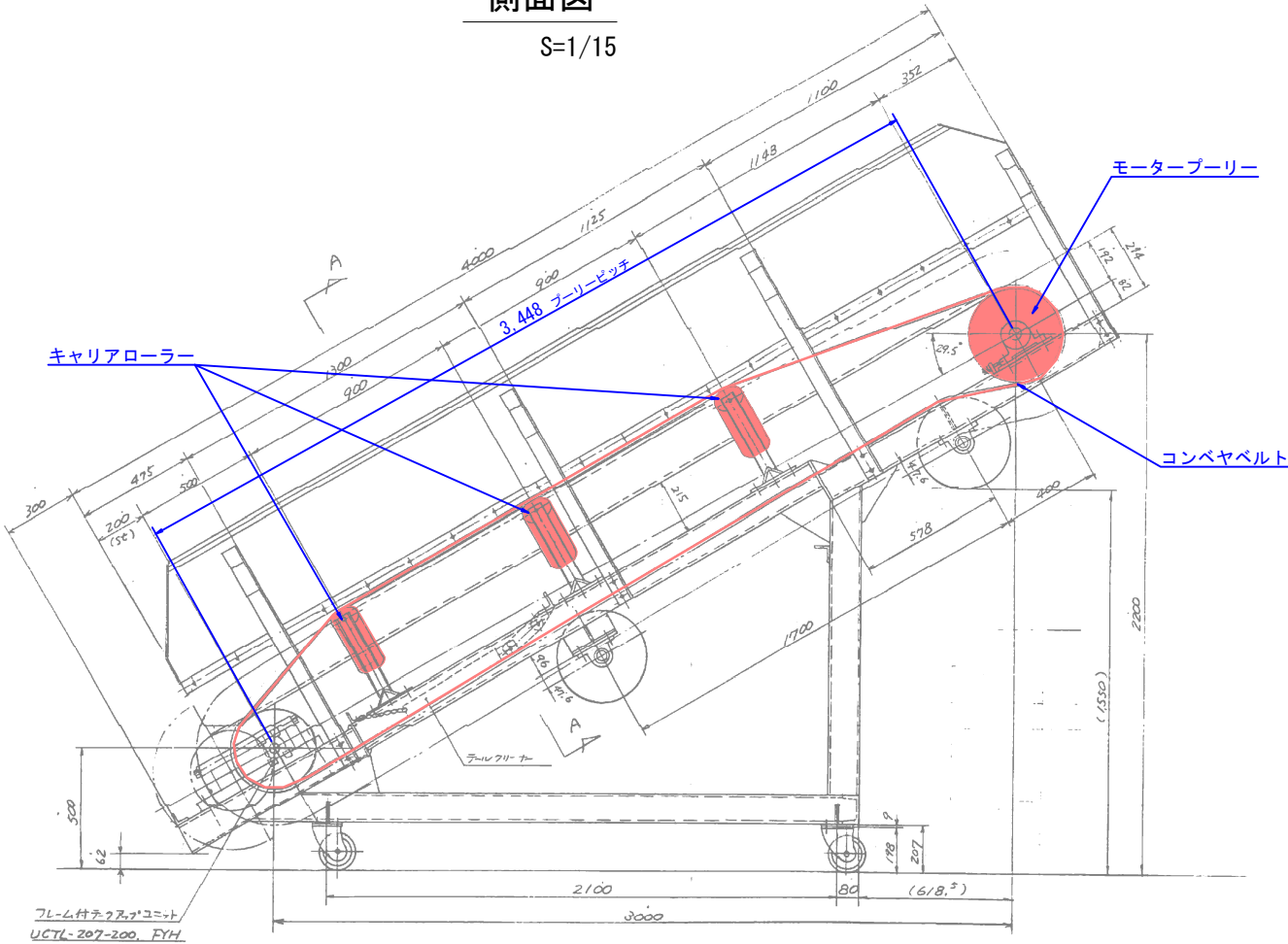
側面図
