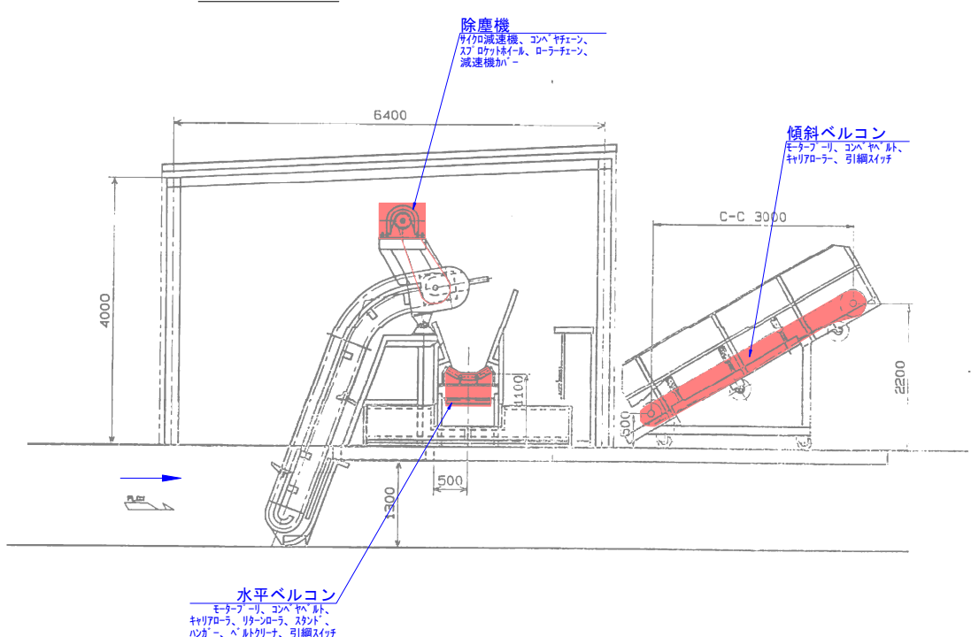
側面図
