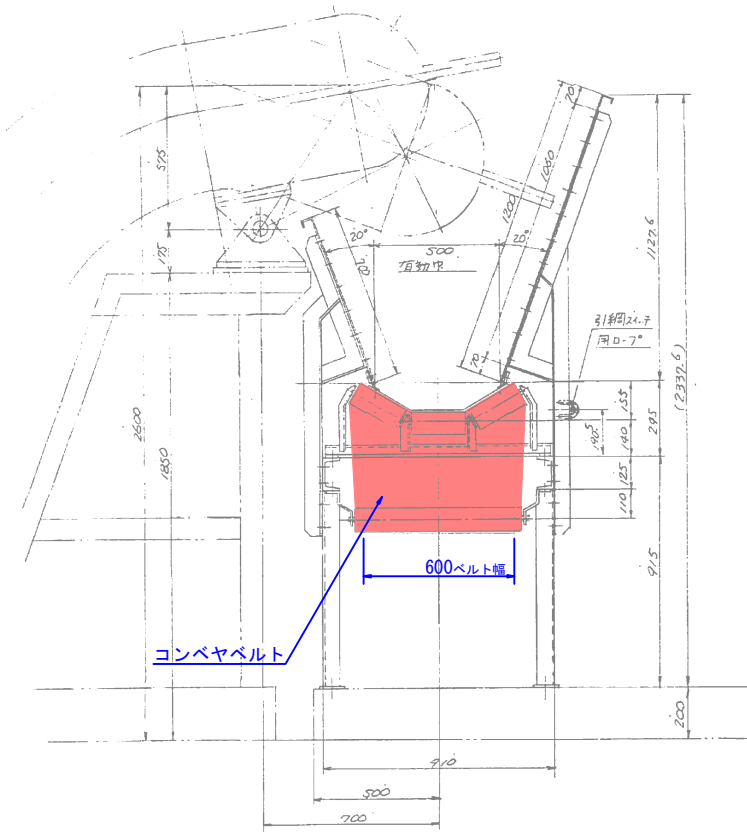
断面図
