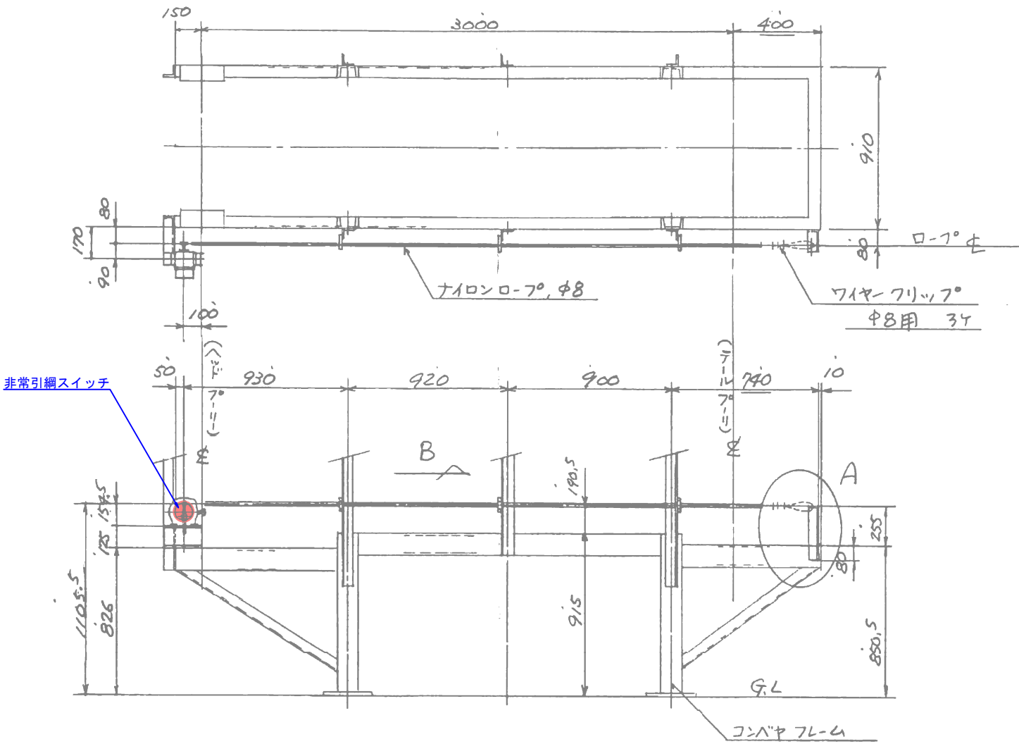
非常引綱スイッチ構造図
