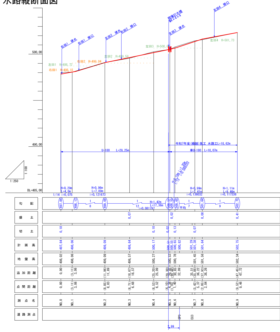
水路縦断面図
