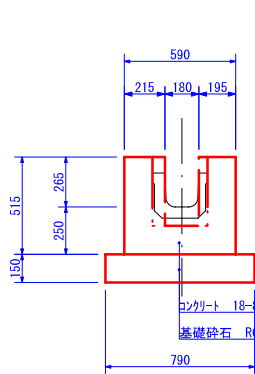
B断面
