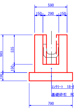
A断面
