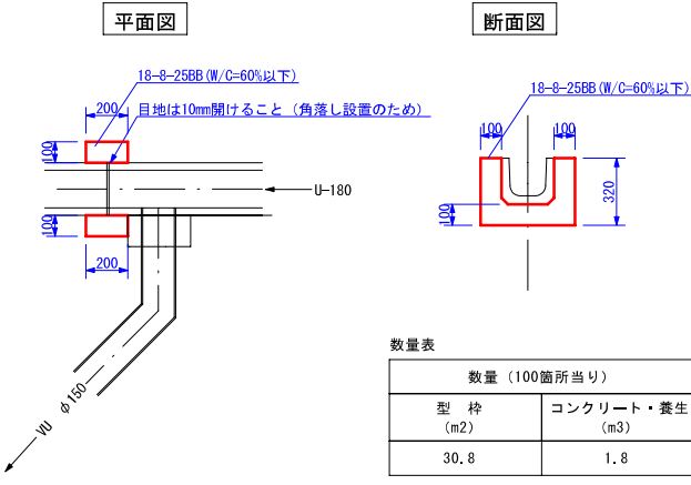
車U-180 巻立工
