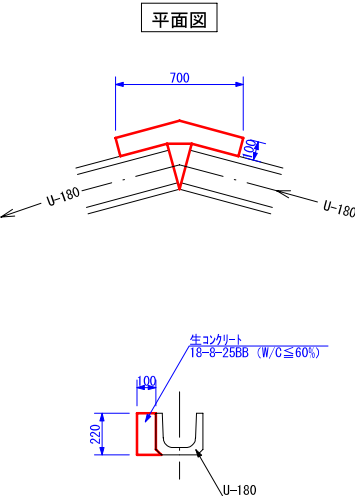
U-180補強工
