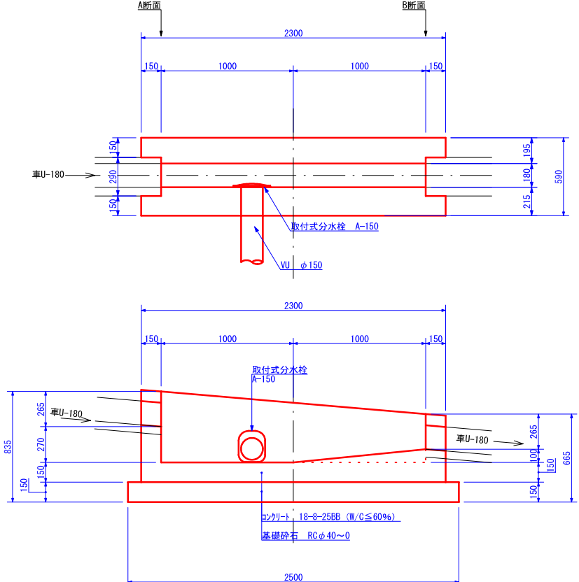
現場打掛口工
