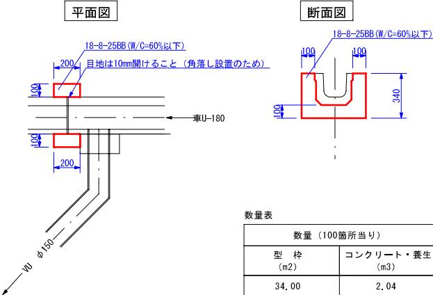
車U-180 巻立工
