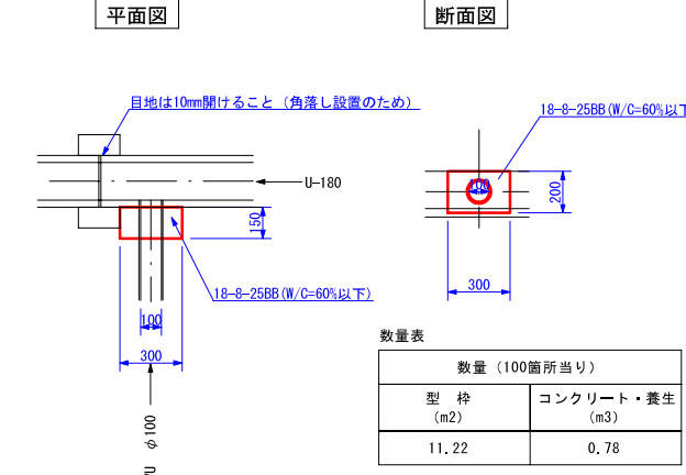
VUφ100 巻立工
