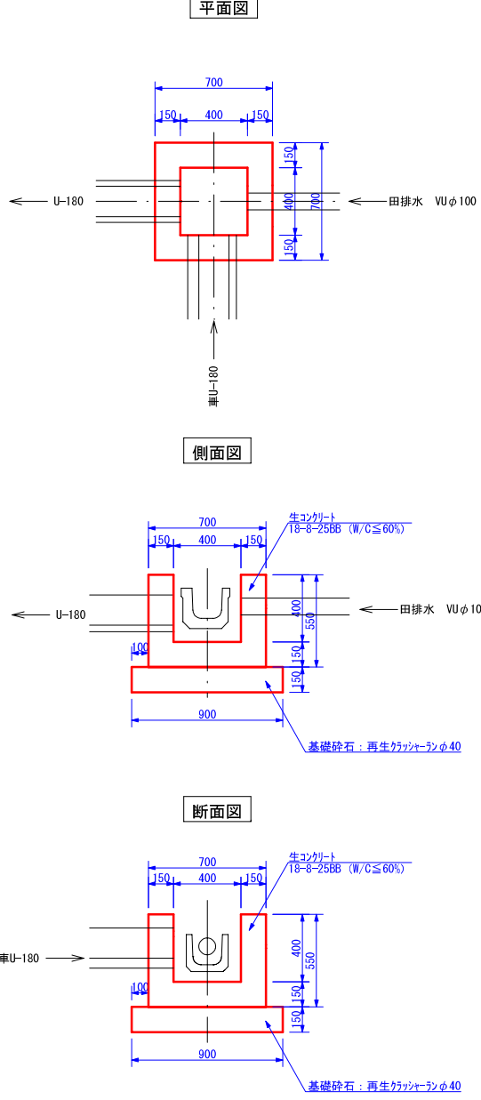
現場打水槽 M4×4×4
