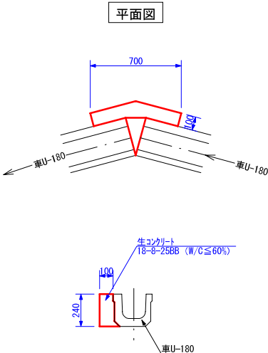
車U-180補強工
