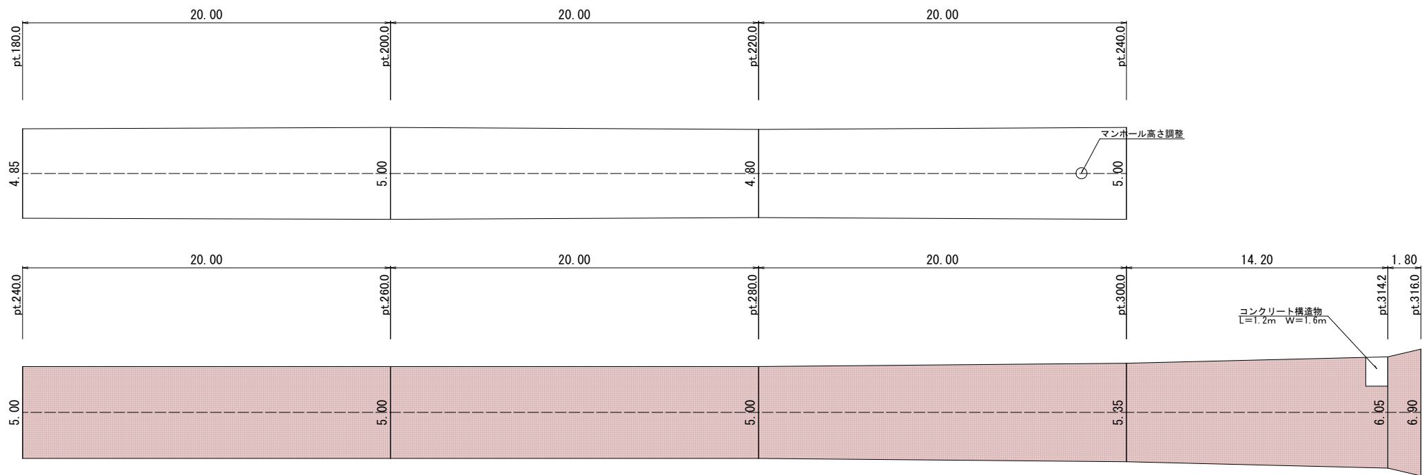
舗装展開図2 S=1:100
