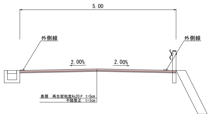
標準横断面図 S=1:25
