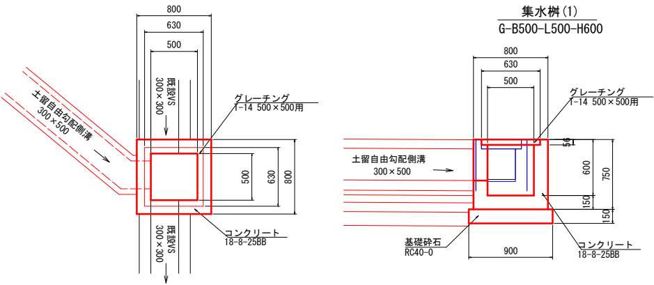
集水枡 (1) 数量表
