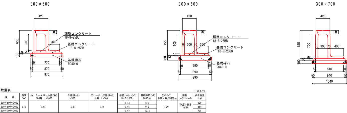
土留自由勾配側溝（センタースリットタイプ） S=1：20
