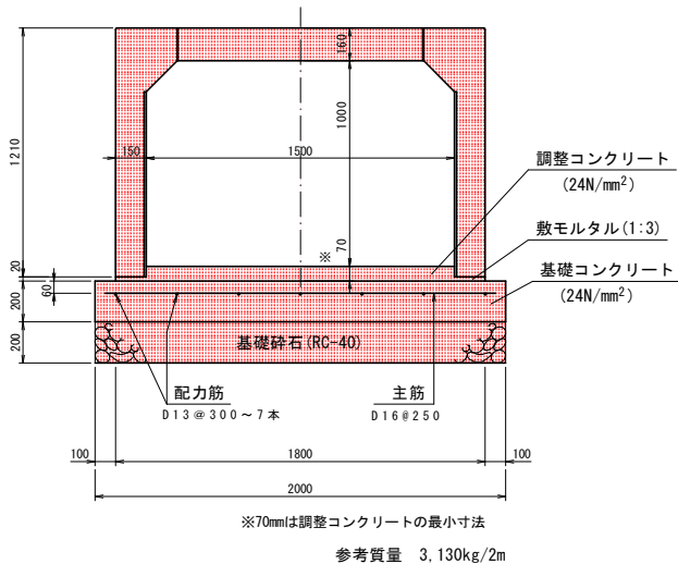
構造図 S=1:20 B1500xH1000 (参考図)
