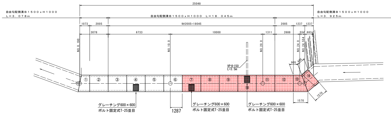
平面割付図 S=1:100 自由勾配側溝 B1500×H1000
