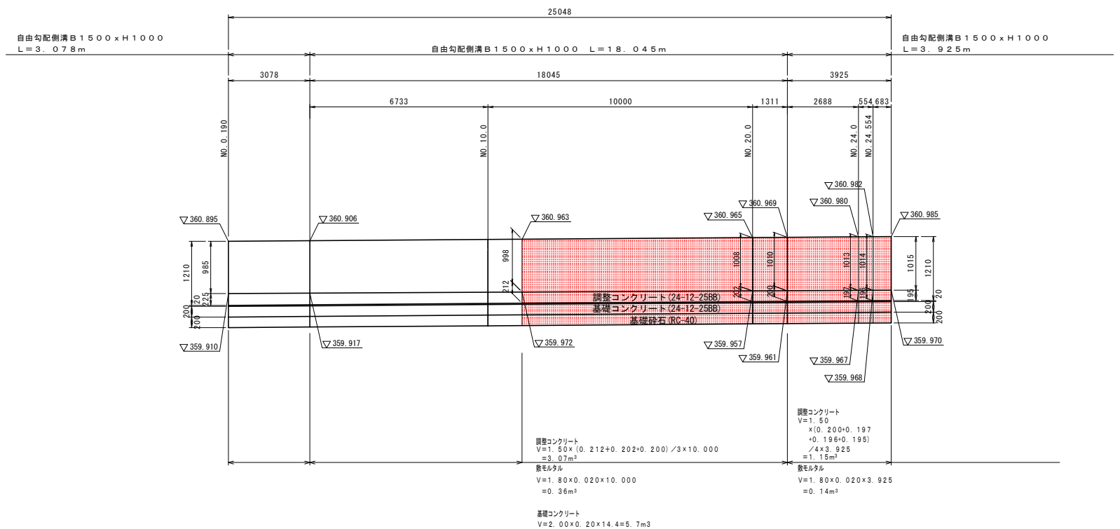
縦断図 V=1:50 H=1:100 自由勾配側溝 B1500×H1000
