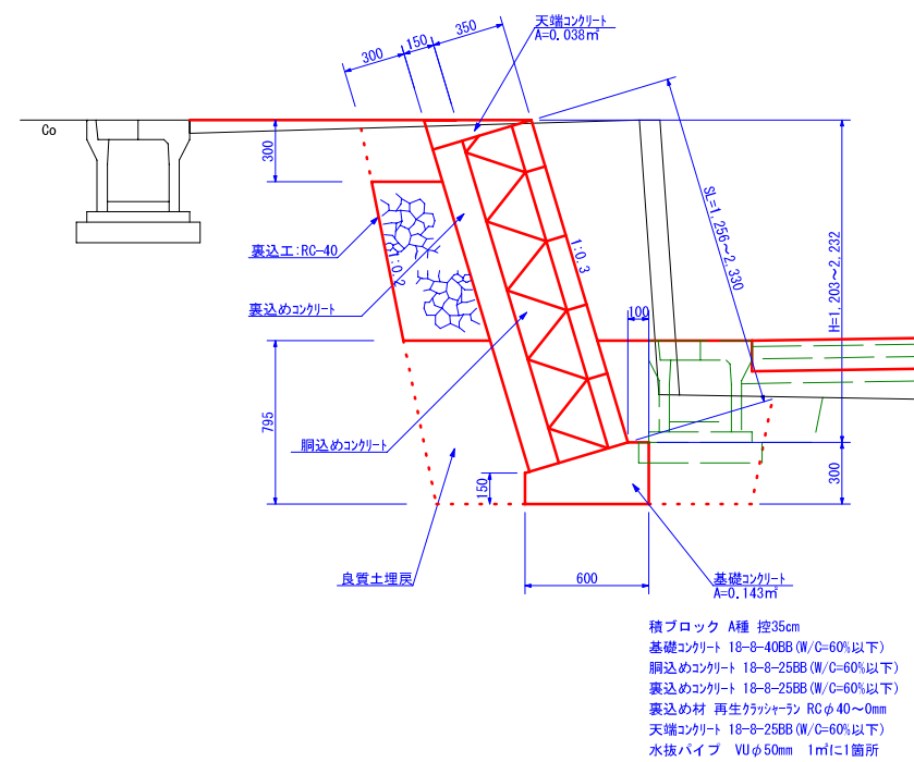
ブロック積工断面図 S=1/20
