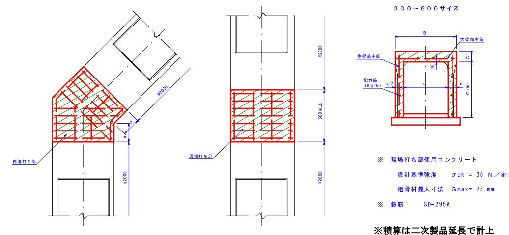
寸法・配筋表（標準部）
