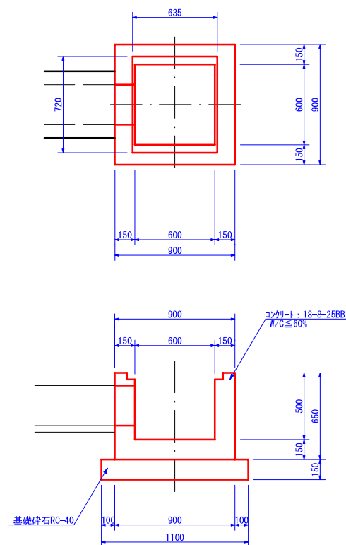
現場打水槽工構造図
