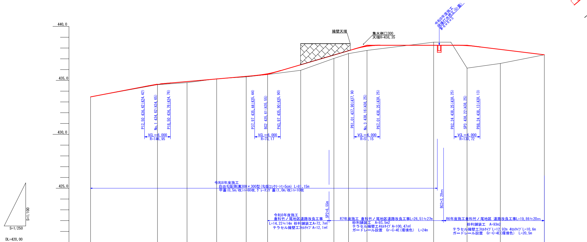
計画縦断面図
