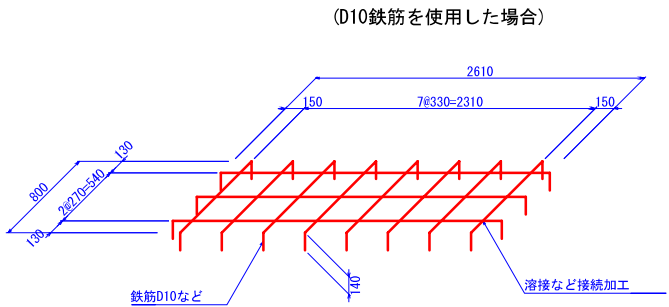
テラセル展開補助枠（3セルタイプ参考）
