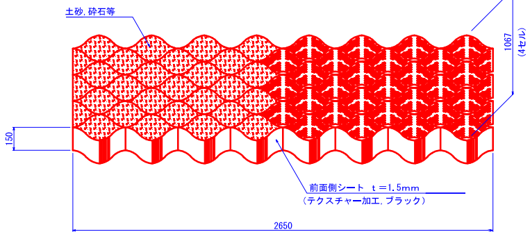
テラセル形状図（4セルタイプ）
