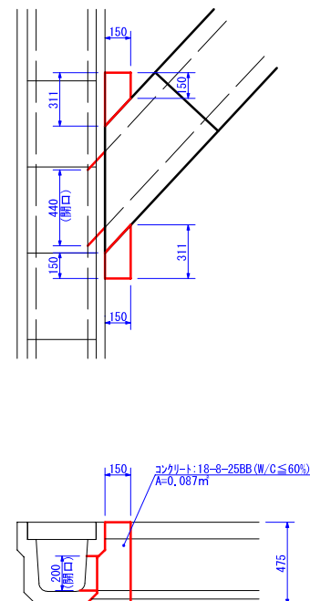
接續部補強工構造図
