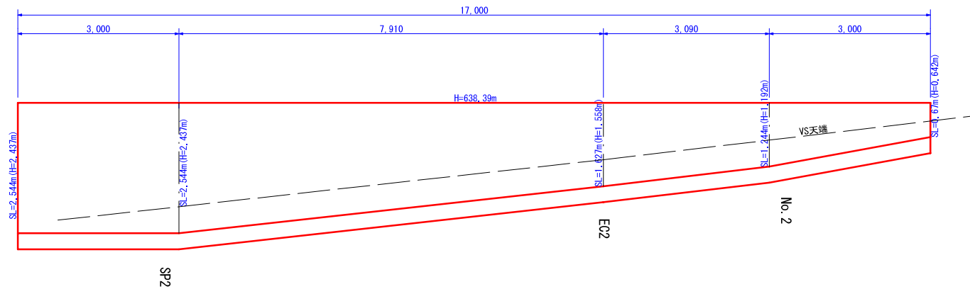
ブロック積工詳細図 S=1/50
