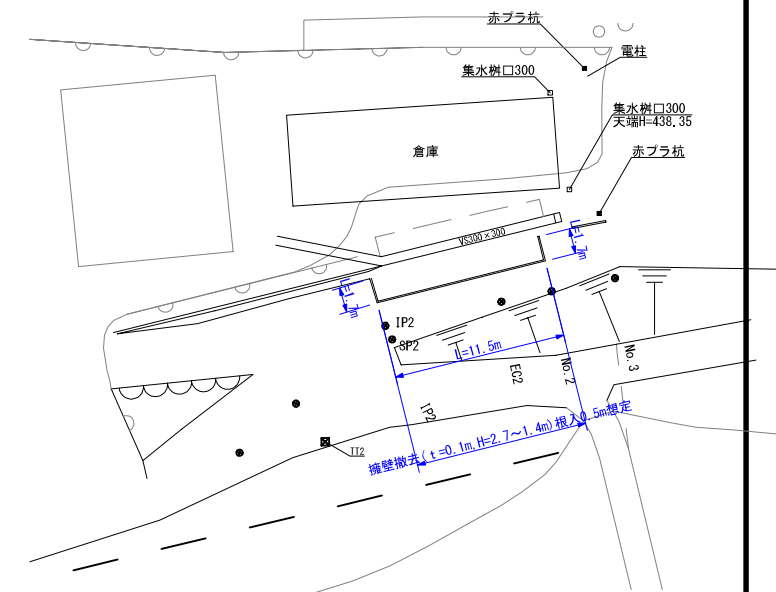
撤去平面図
