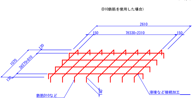
テラセル展開補助枠（4セルタイプ参考）
