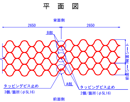
テラセル相互接合部詳細
