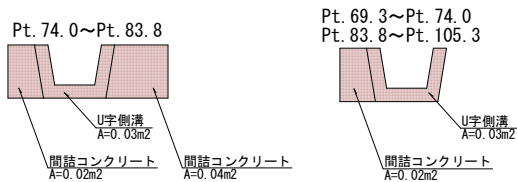
間詰コンクリート及びU字側溝
