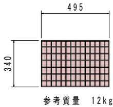
グレーチング蓋（参考図）
