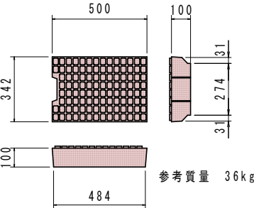
コンクリート蓋（参考図）
