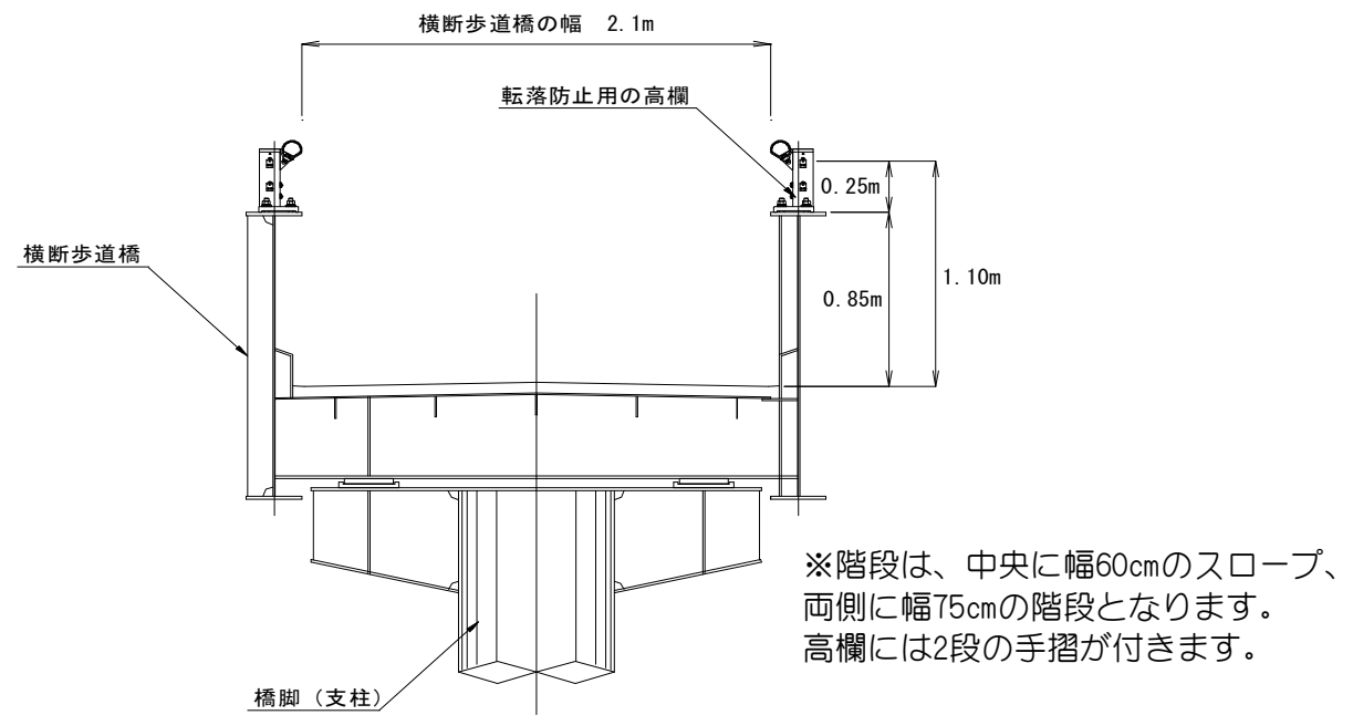
歩道橋の断面図
