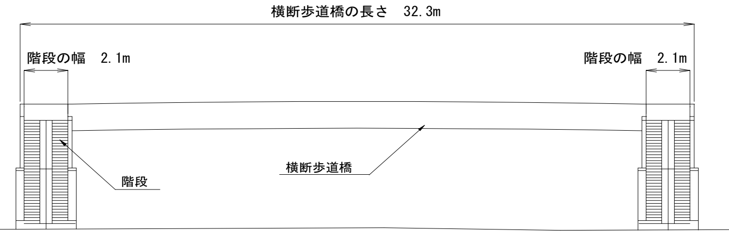
歩道橋の断面図
