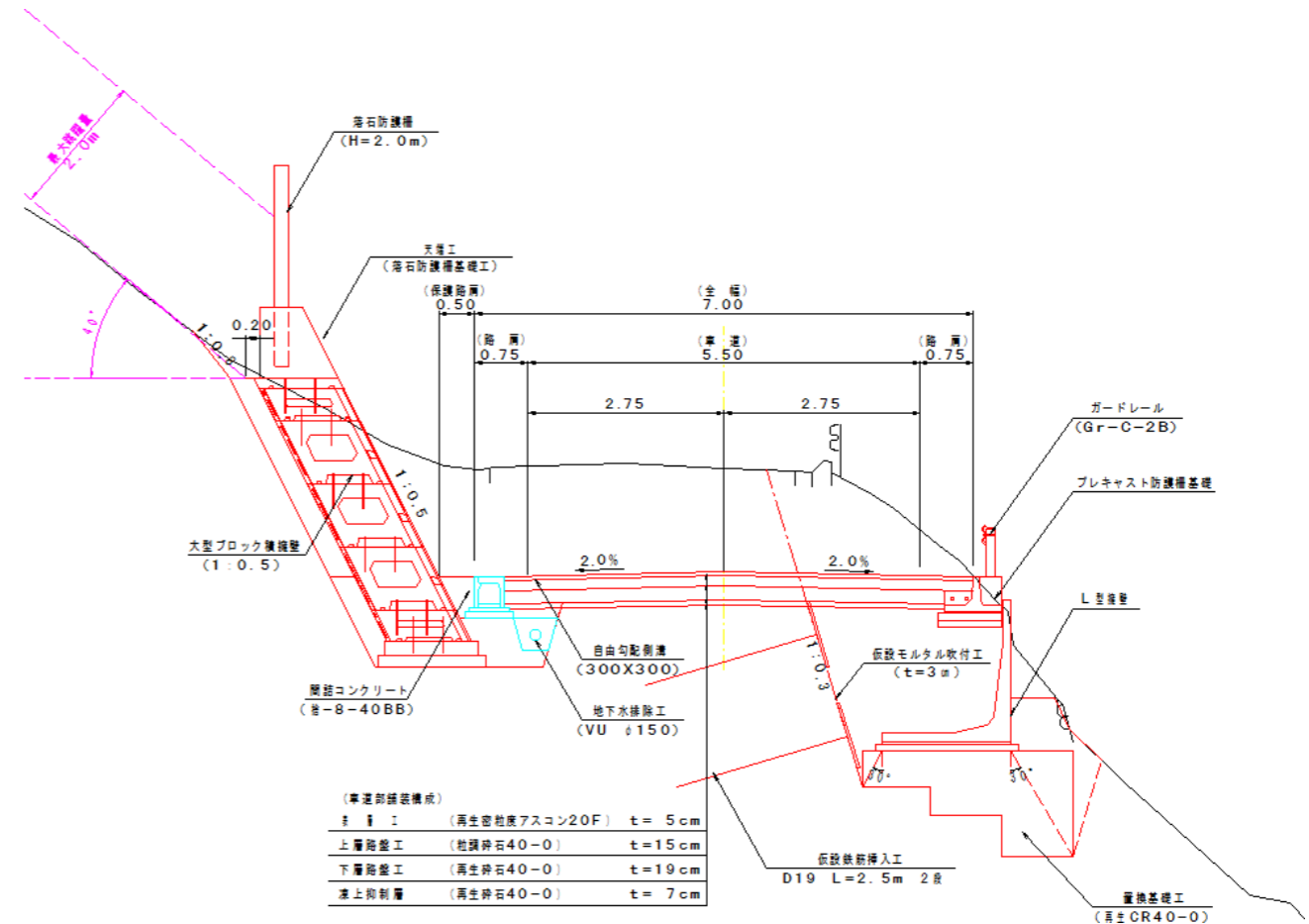
— 標準横断図 —
