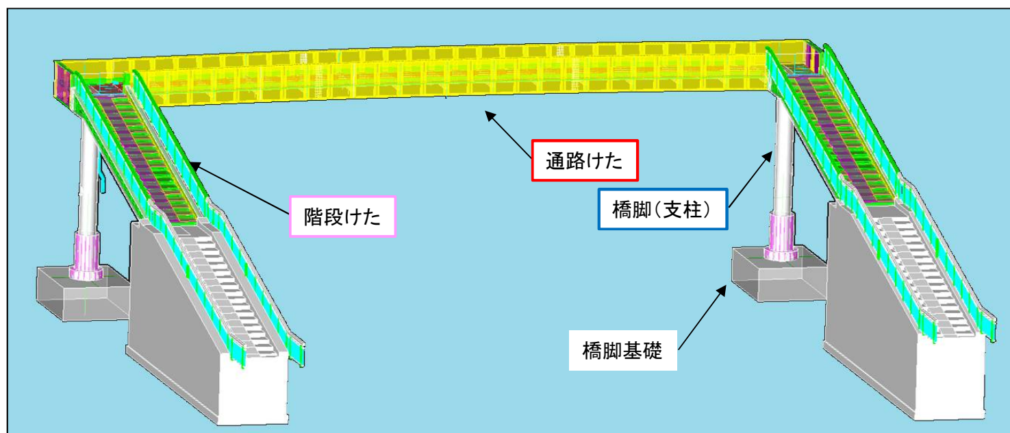
横断歩道橋の完成モデル
