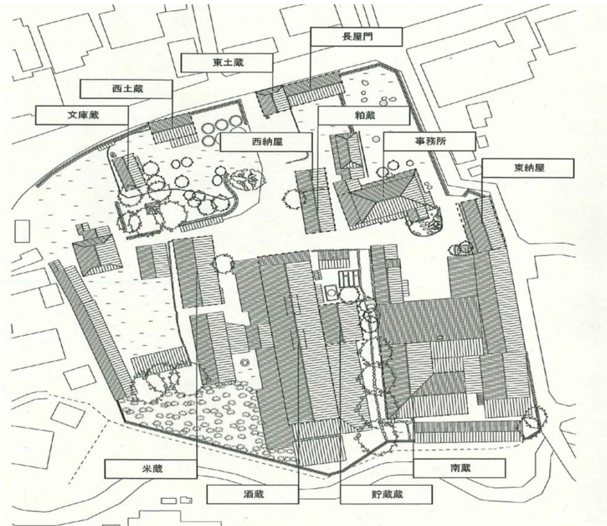
長野銘醸(和田酒店)建物配置
