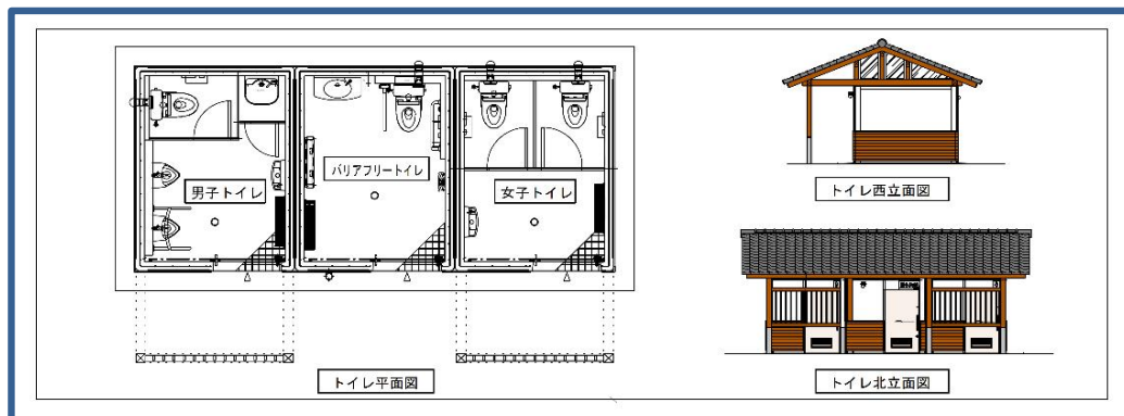
公衆トイレ(案)
