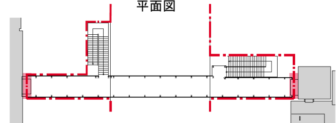
平面図
