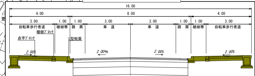
現況断面図
