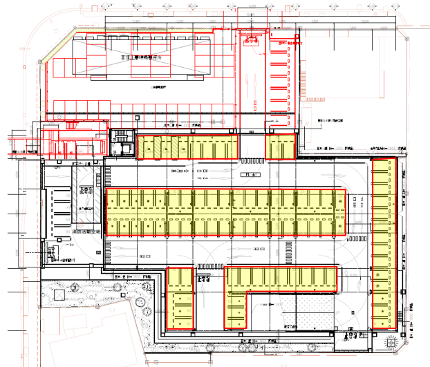
1階平面図 (78台)
