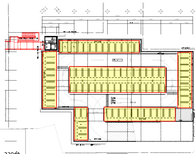
R階平面図 (75台)
