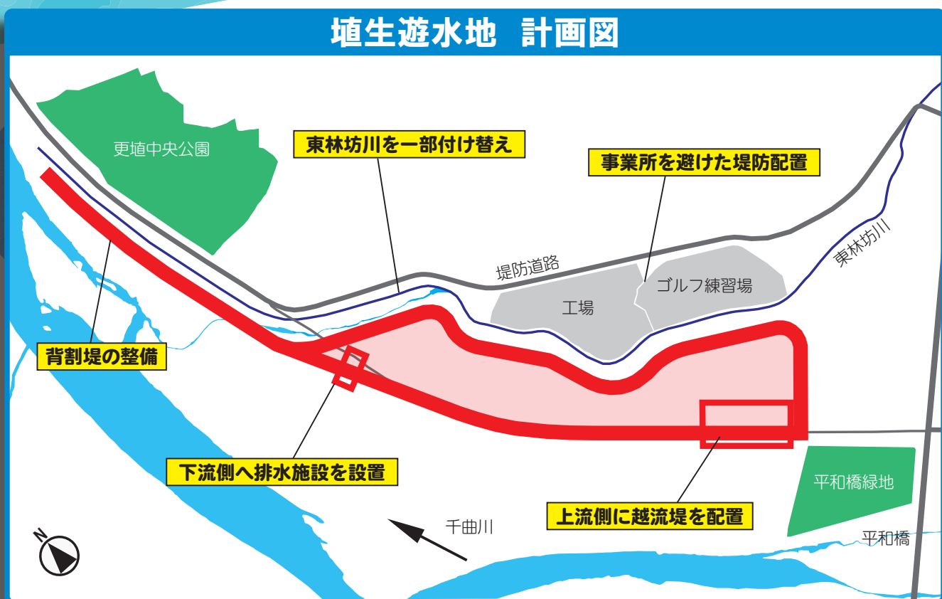
平和橋遊水地 計画図
