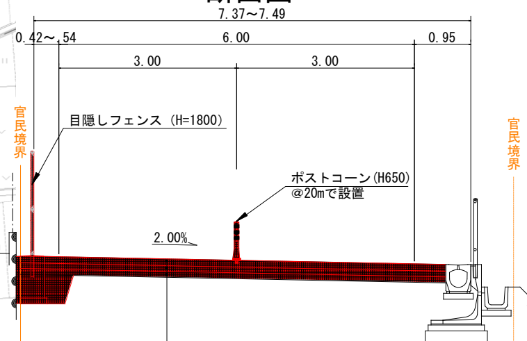
断面図
