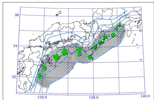
(図-3) 南海トラフ巨大地震の断層モデル 内閣府 (2012) (上図：基本ケース、下図：陸型ケース)
